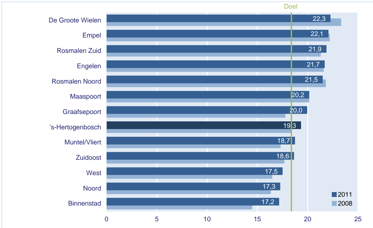
Afbeelding 3: Veiligheidsindex wijken (2008-2011)
